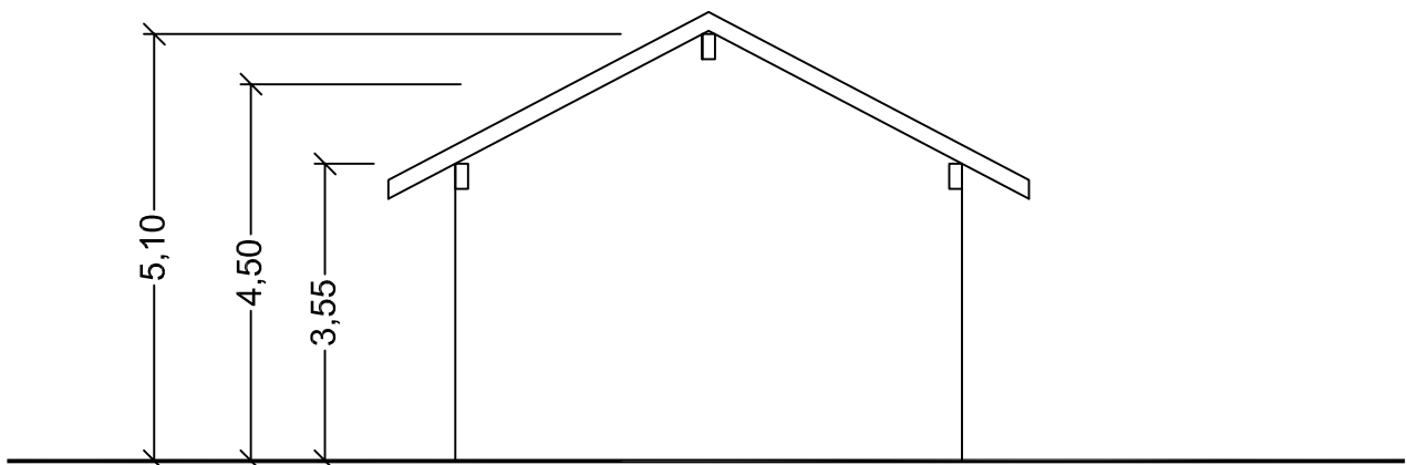
prospetto 1:100
