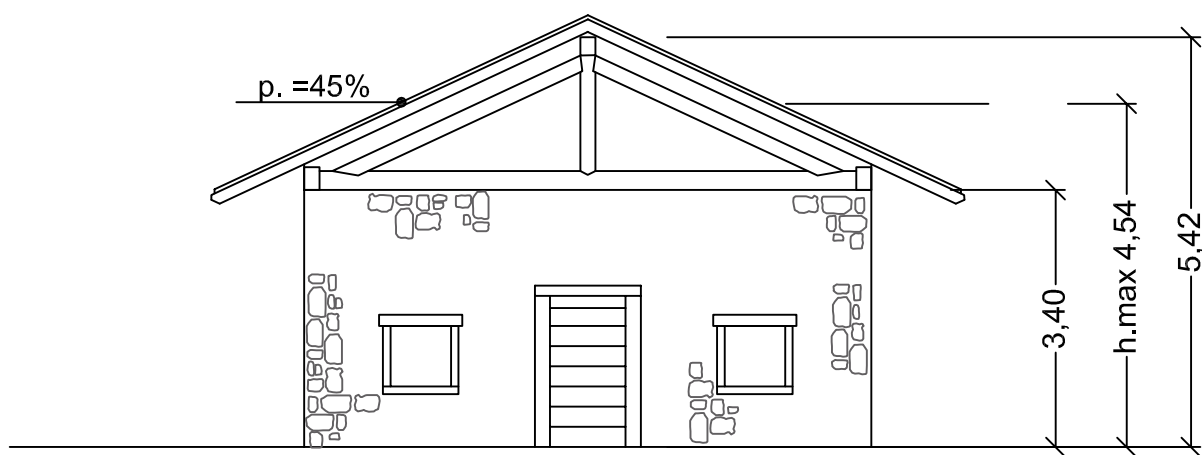
prospetto 1:100
