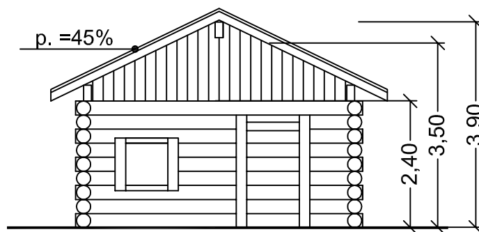
prospetto 1:100
