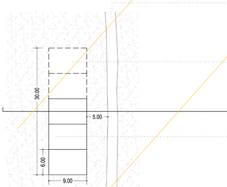
PIANTA scala 1: 500
