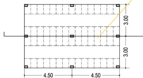
PIANTA
