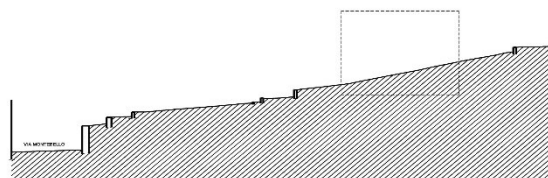
SEZIONE A-A' STATO ATTUALE scala 1:250
