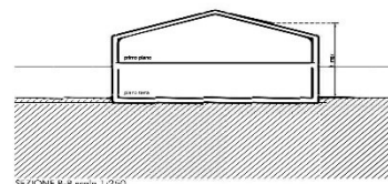
SEZIONE B-B' scala 1:250
